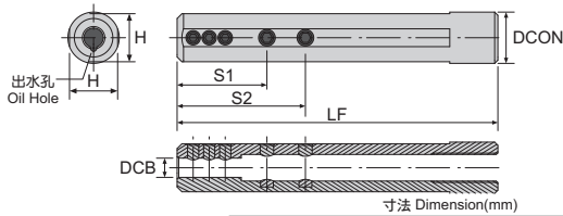
寸法 Dimension(mm)
